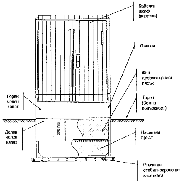
фигура – Монтаж на пластмасов разпределителен шкаф (касета)
