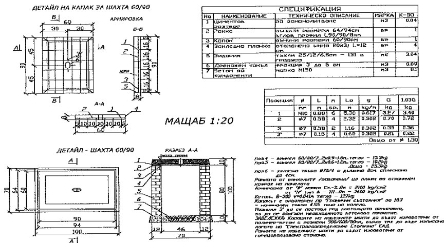
Фиг.6.3. Кабелна шахта – единична
